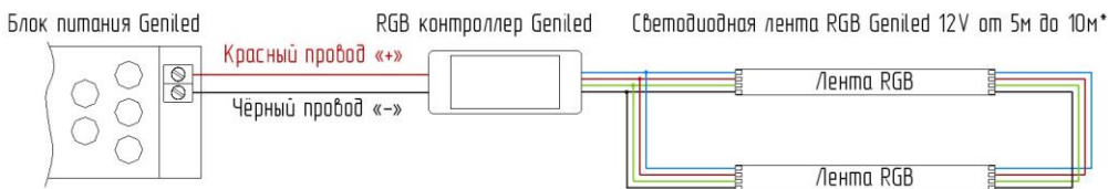
Рисунок 6. Пример подключения ленты Geniled RGB от 5м до 10м.
